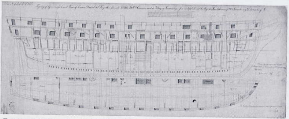
Fregatten Gefjon : Tegning fra Rigsarkivet, Søetatens tegningsamling. Det var denne fregat Claus Clausen var ombord på i 1848.
